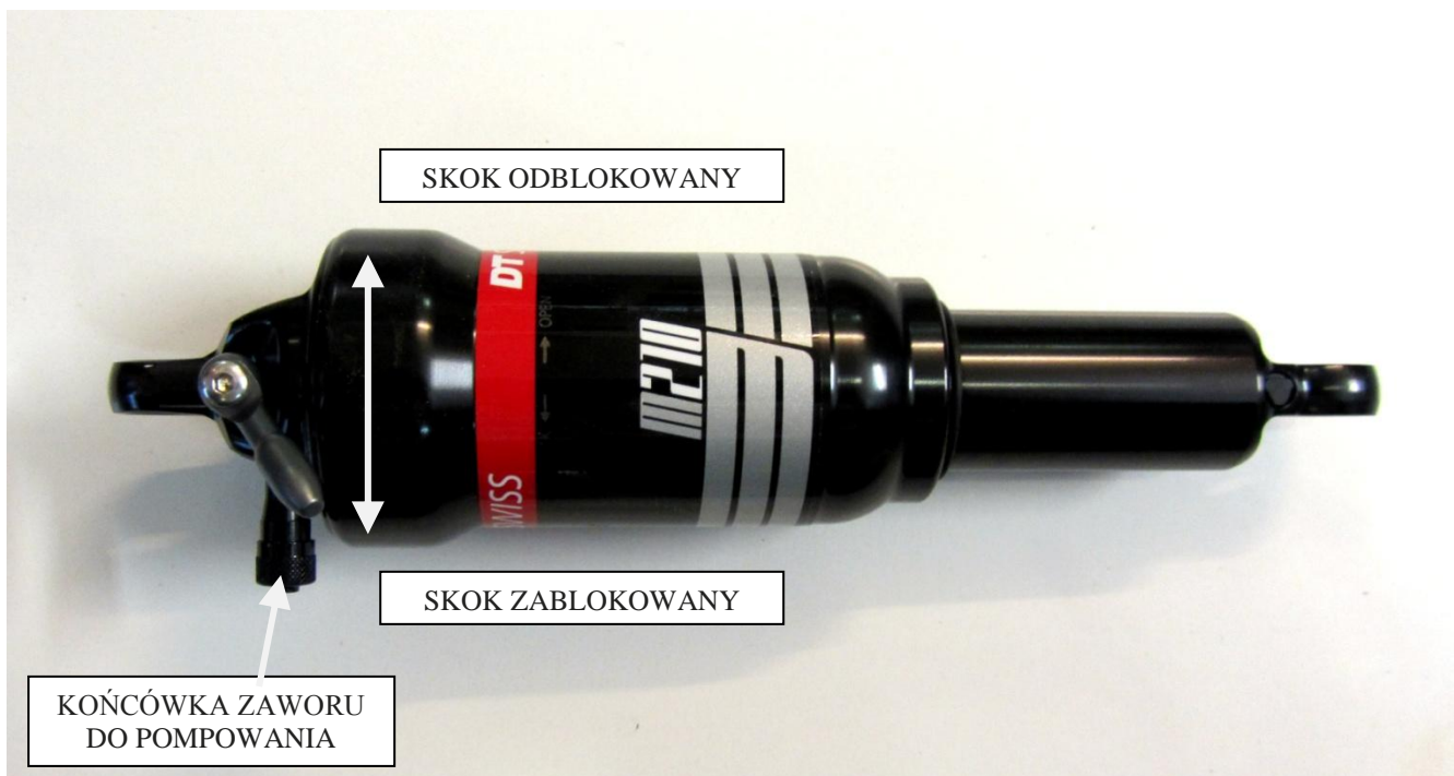
Rys. 16 Regulacja amortyzatora
