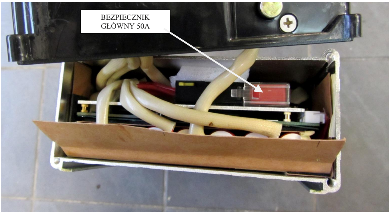
RYS. 13B BEZPIECZNIK GŁÓWNY
