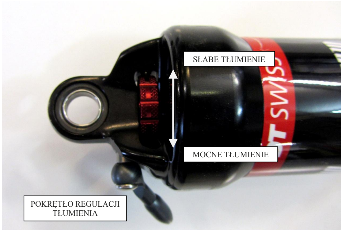
Rys. 15 Regulacja amortyzatora
