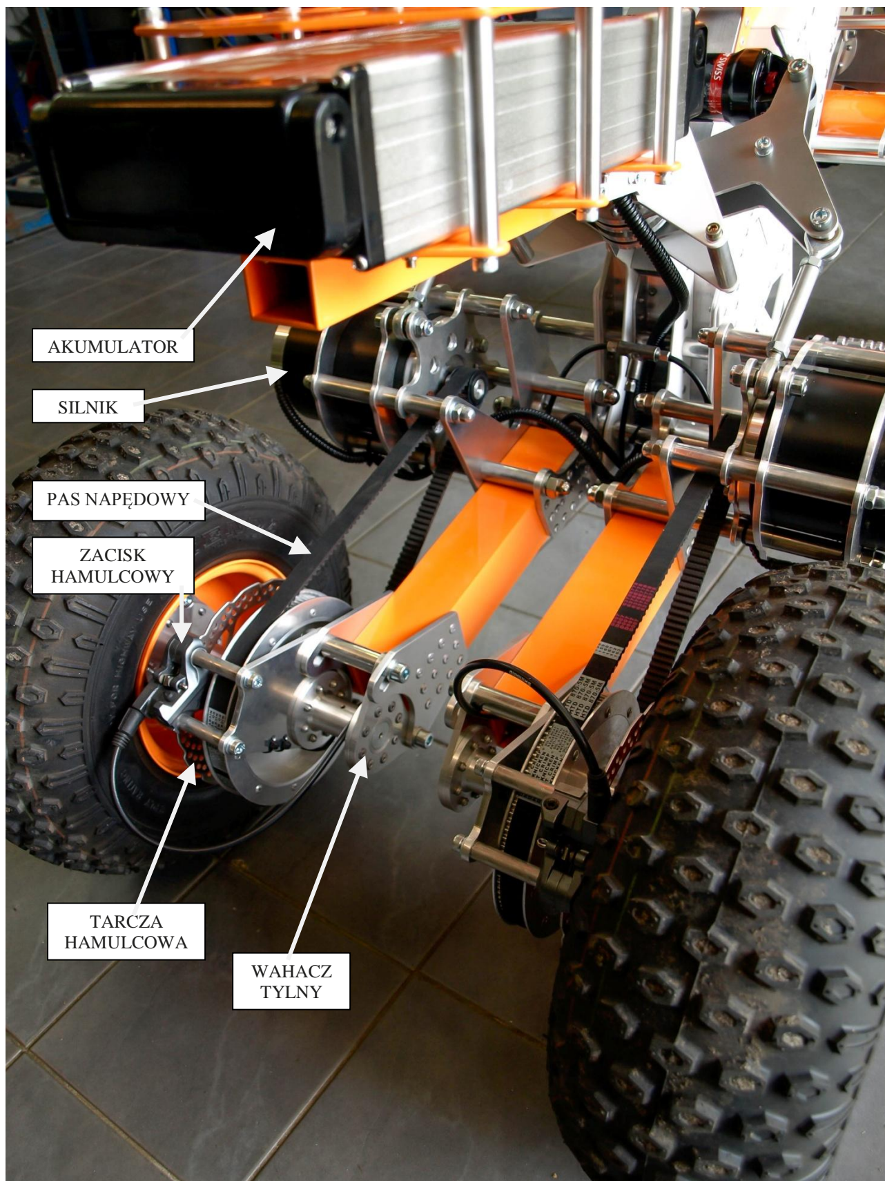
Rys. 2 CZĘŚCI SKŁADOWE
