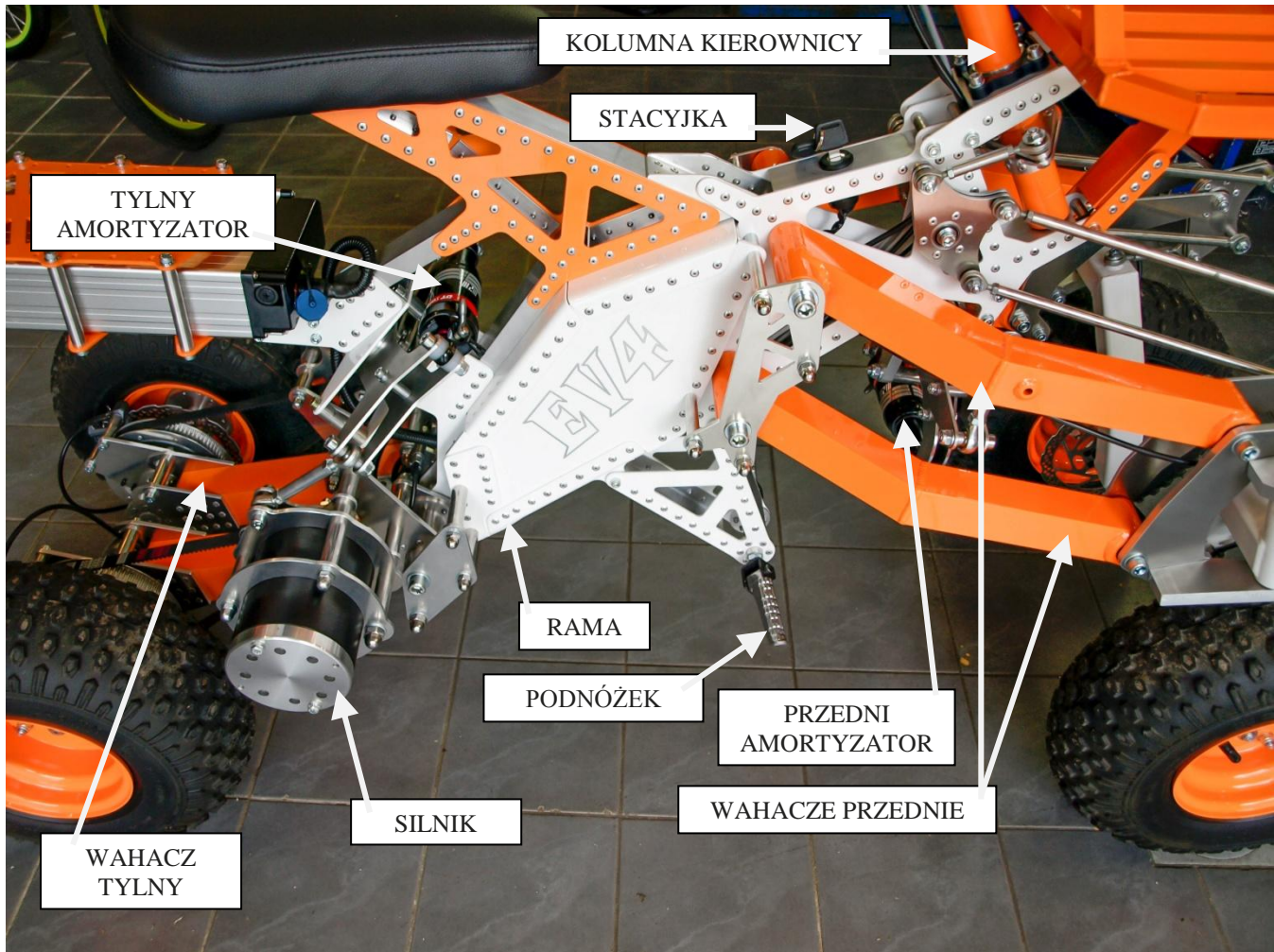
Rys. 4 CZĘŚCI SKŁADOWE
