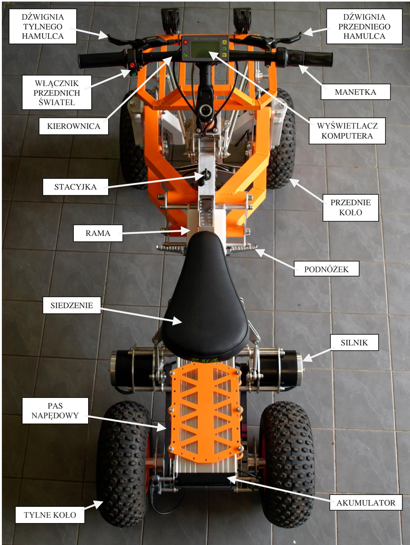
Rys. 8 CZĘŚCI SKŁADOWE
