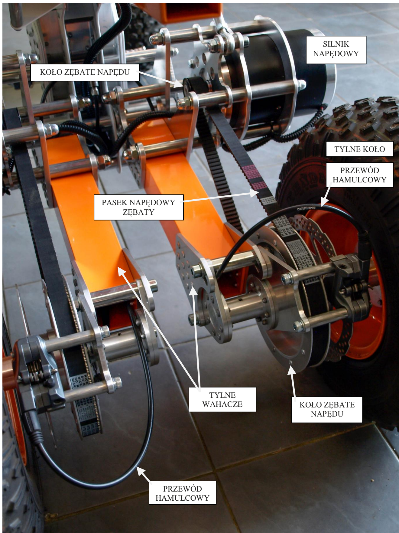
Rys. 5 CZĘŚCI SKŁADOWE
