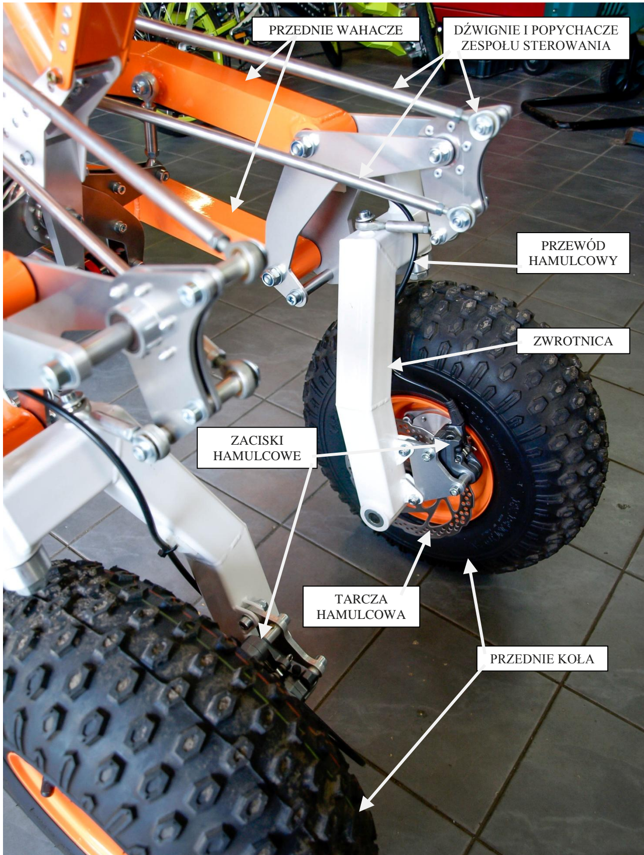
Rys. 3 CZĘŚCI SKŁADOWE
