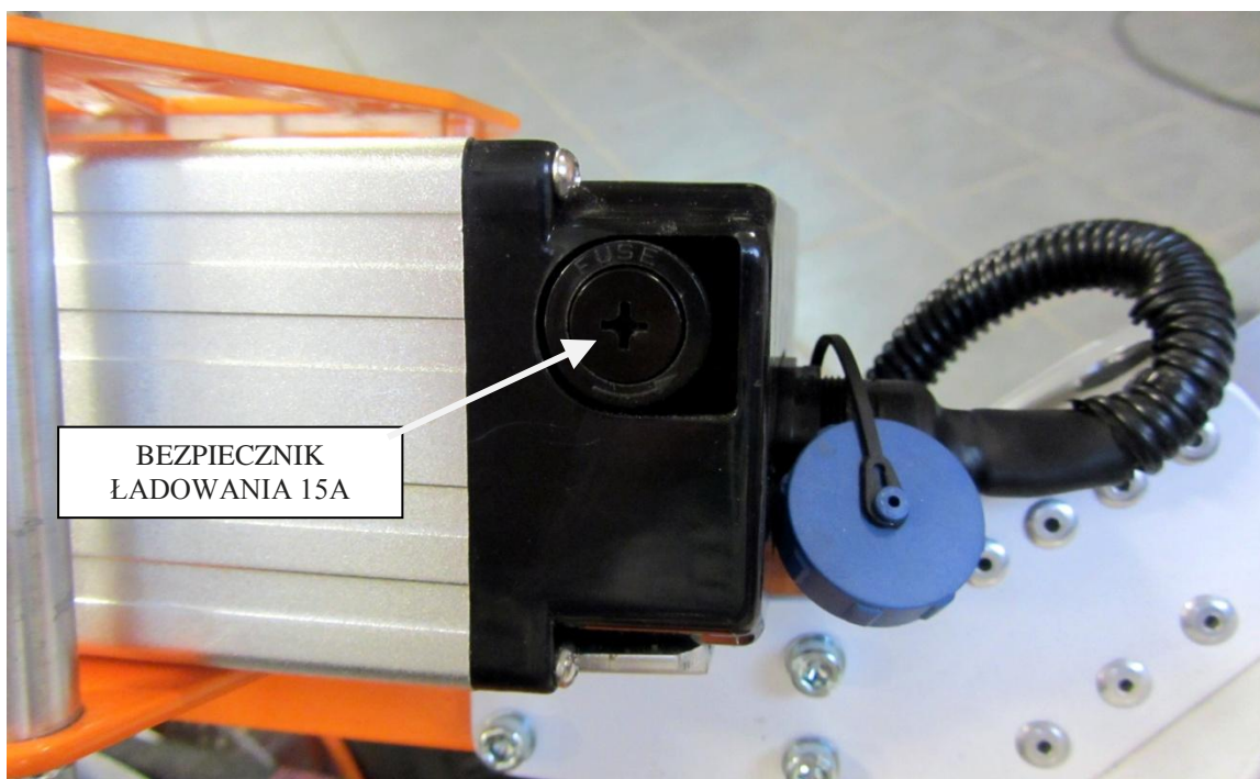
RYS. 13 BEZPIECZNIK ŁADOWANIA
